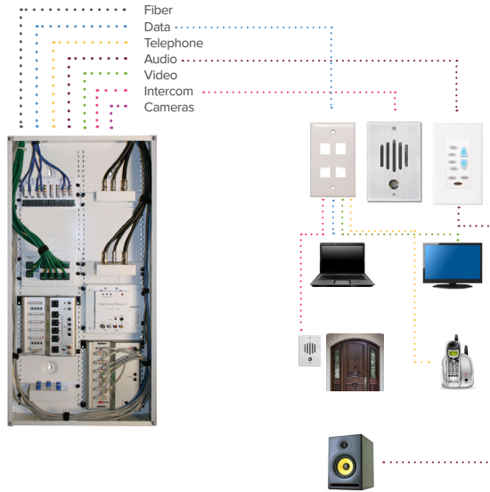
12" Enclosure ■ C-0112E
